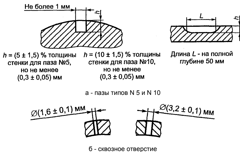
Рисунок В.1. Виды искусственных дефектов (рисунок В.1 в ред. Изменения N 1, утв. Приказом Ростехрегулирования от 24.08.2007 N 213-ст)
