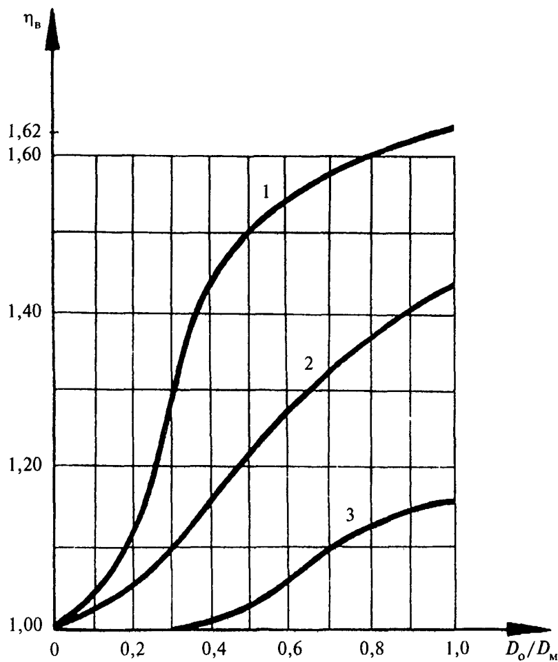
ГРАФИК ДЛЯ ОПРЕДЕЛЕНИЯ КОЭФФИЦИЕНТА НЕСУЩЕЙ СПОСОБНОСТИ ТРОЙНИКОВ \eta_v
