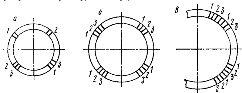
Рис. 3. Схема вырезки образцов для механических испытаний
