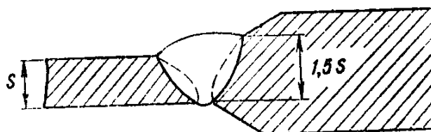
Рис. 2. Подготовка промок патрубков арматуры при непосредственном соединении их с трубами
