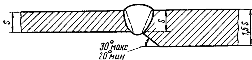
Рис. 1. Конструктивные размеры разделки кромок и сварных швов разнотолщинных труб (до 1,5 толщины стенки)
